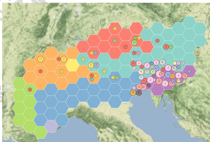
Figura 1: Mappa interattiva
